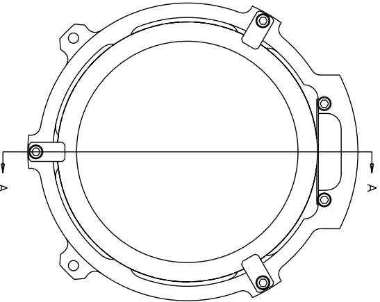
FRONT: SCALE 1:1
