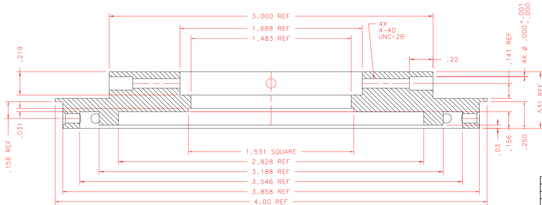
SECTION A-A SCALE 2:1
