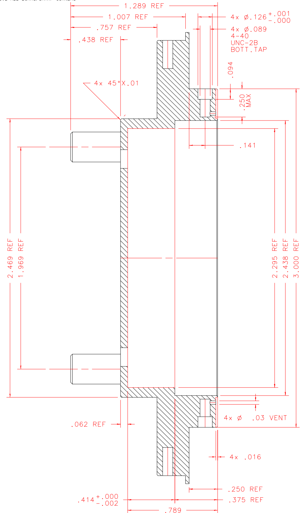
SECTION A-A: SCALE 2:1
