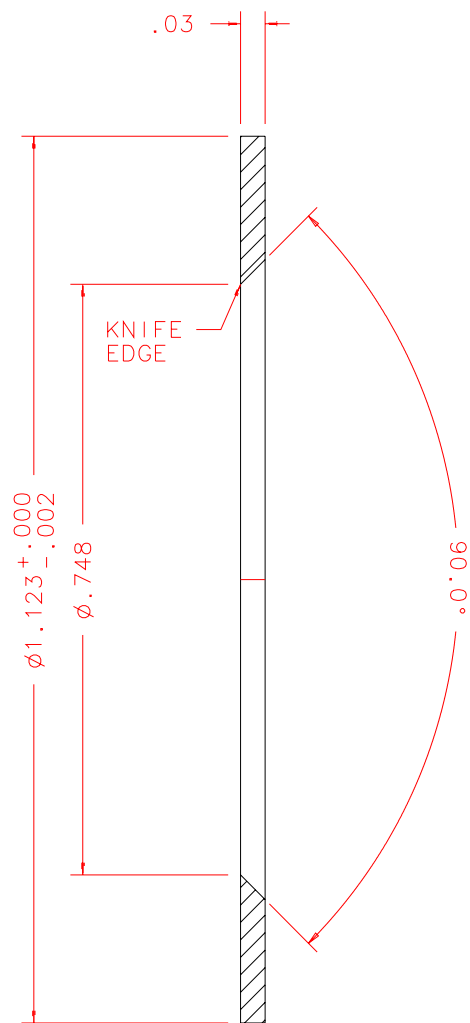
SECTION A-A SCALE 4:1
