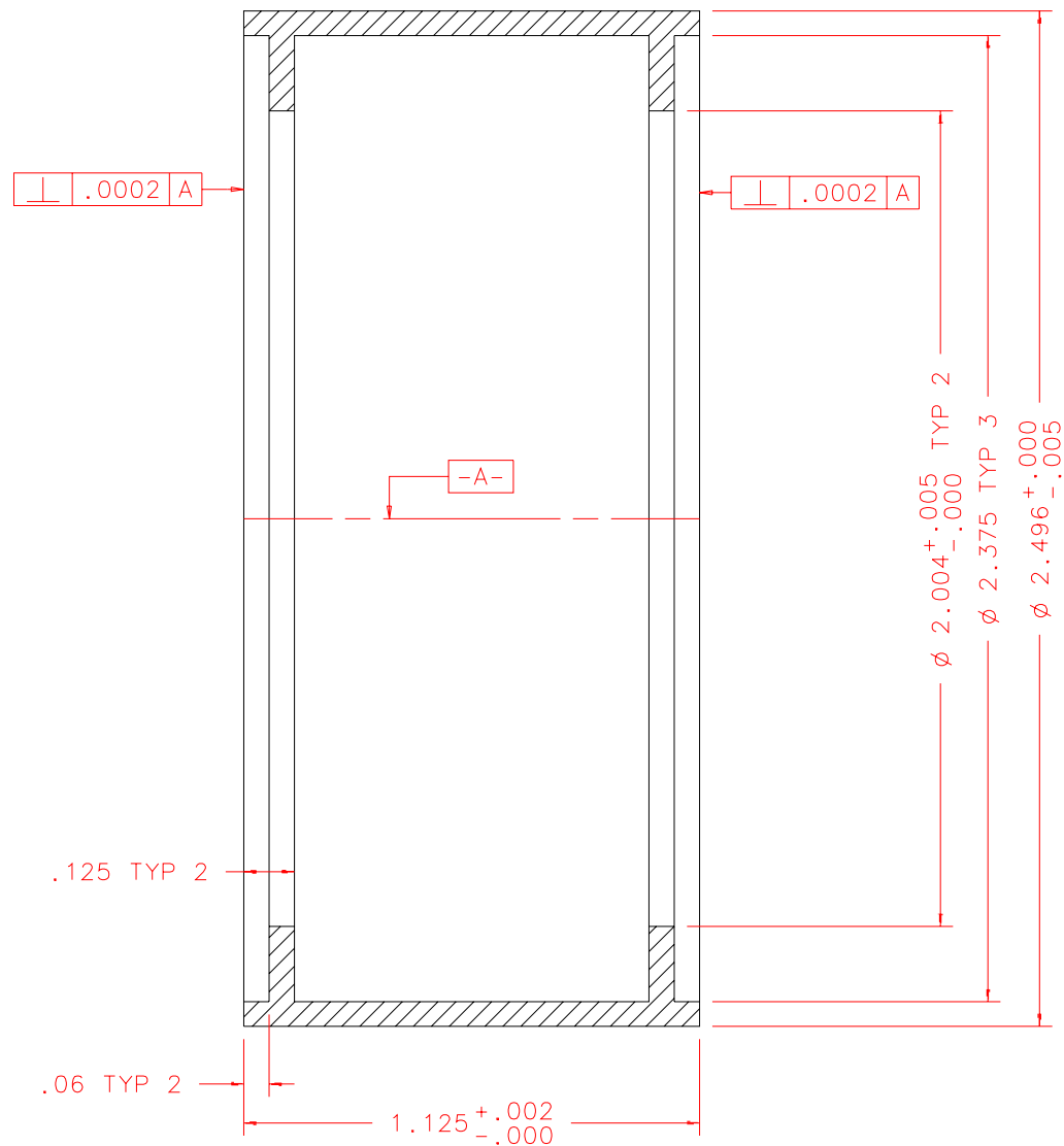
SECTION A-A: SCALE 2:1
