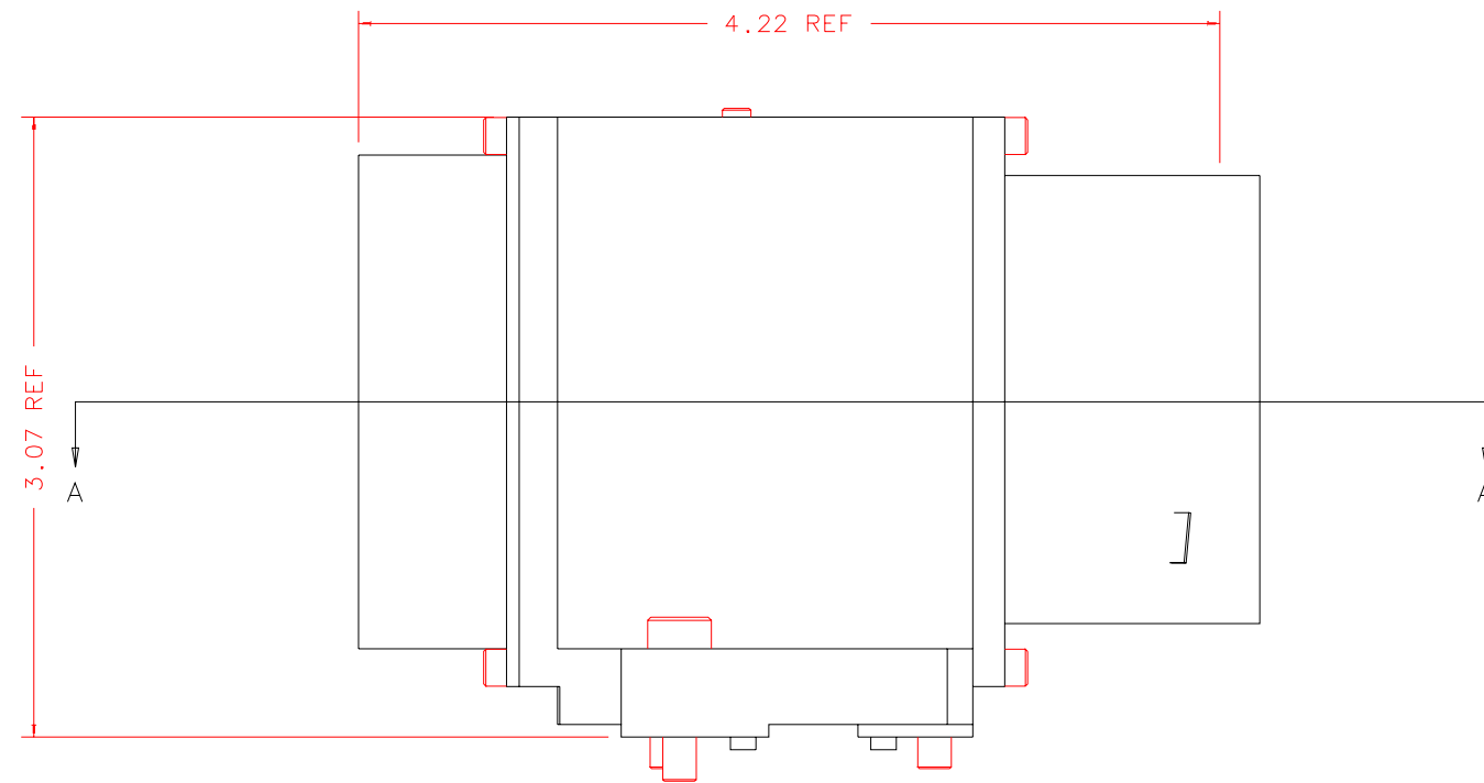
FRONT: SCALE 1:1
