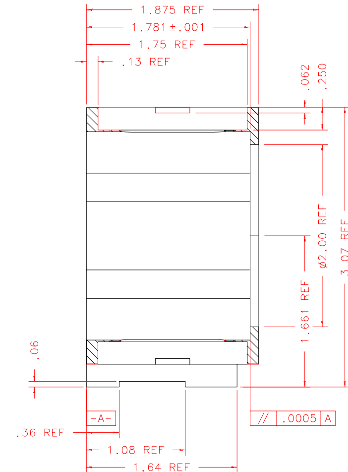
SECTION A-A
