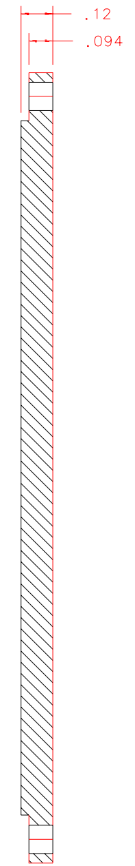
SECTION A-A
