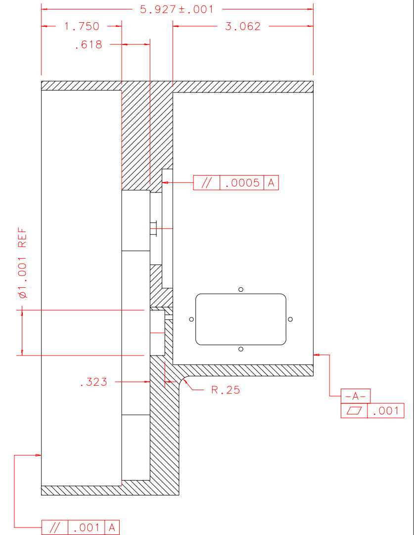
SECTION A-A: SCALE 1:2
