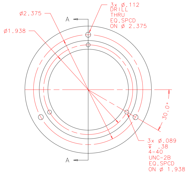
FRONT: SCALE 1:1
