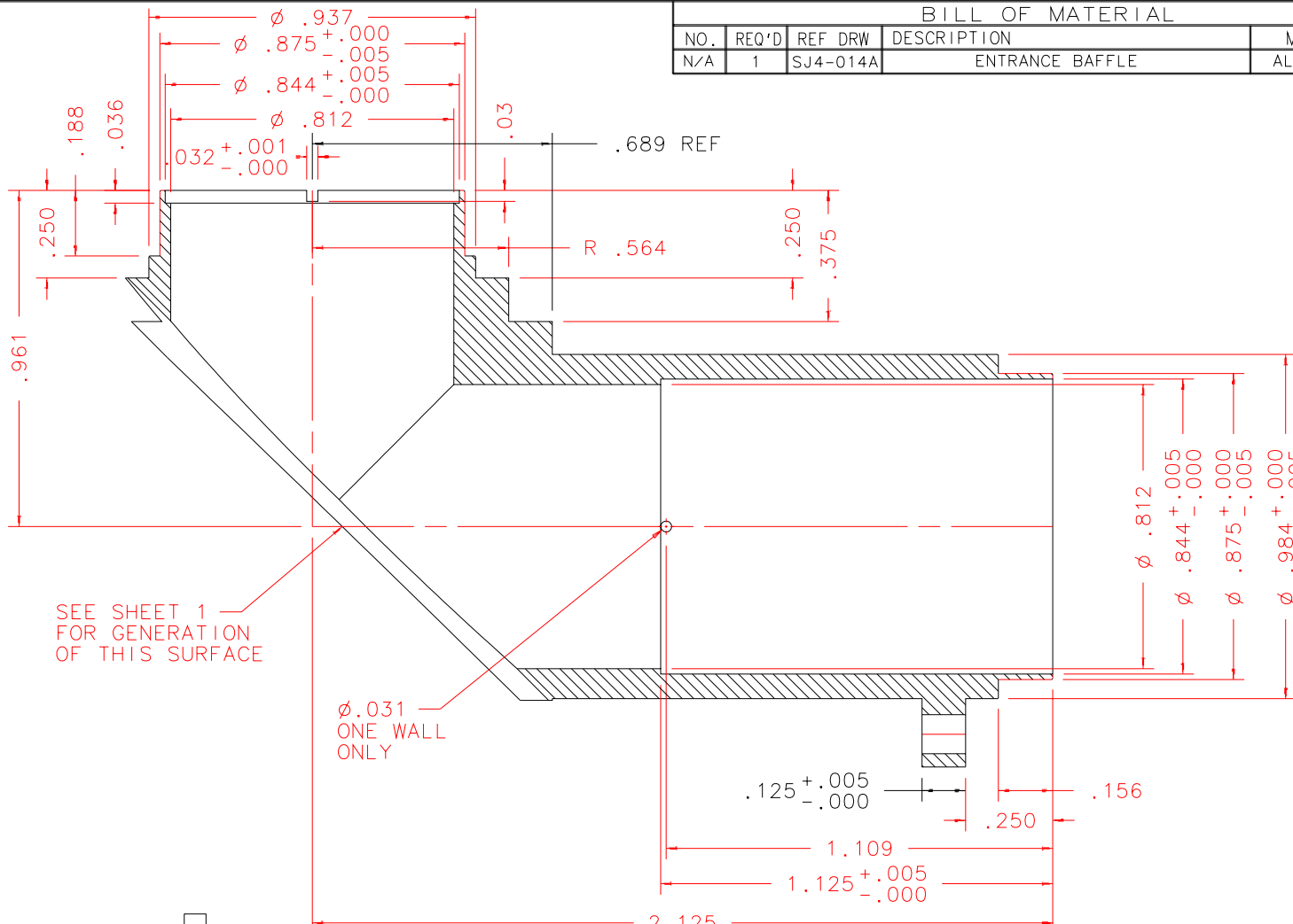
SECTION A-A: SCALE 2:1
