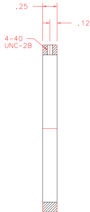
SECTION A-A
