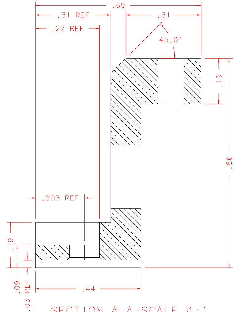
SECTION A-A: SCALE 4:1
